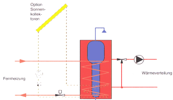
Fernheizungs-Hausstation mit Swiss Solartank ® , Wassererwärmer und Wärmetauscher integriert
